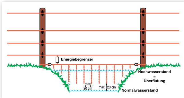
Abbildung 8: Vertikaler Drahtvorhang am Beispiel einer Grabenüberquerung (© links: G. Herkert, © rechts: H. Schumann)
