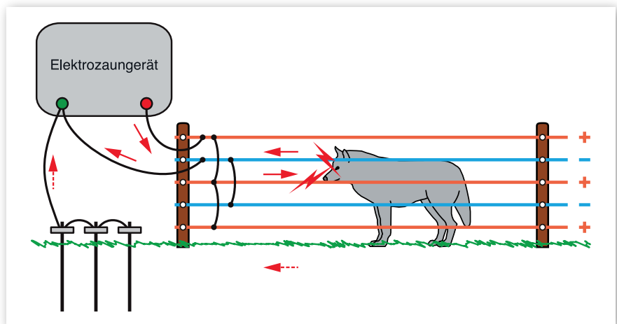
Abbildung 20: Prinzip Plus-Minus-Zaun (© G. Herkert)
