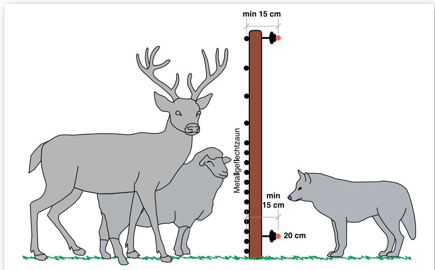
Abbildung 19: Absicherung eines Stabilzäunes mit zwei stromführenden Leitern (© G. Herkert)
