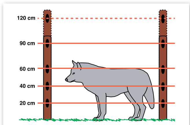
Abbildung 7: Grundaufbau Wolfsabwehrzaun (© G. Herkert)
